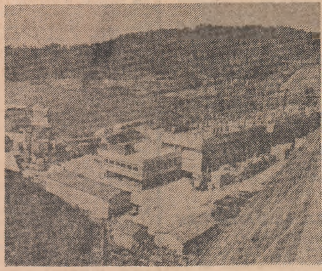
Imagine a complexului hidroenergetic de pe fluviul Nam Ngum
