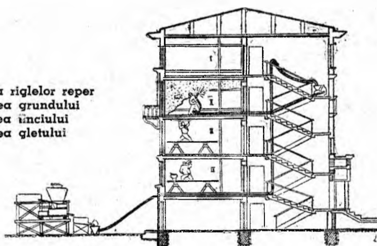
Organizarea lucrărilor de tencuieală mecanizate după metoda În lanț
