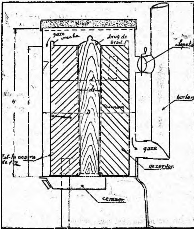
Detalii de construcție a sobei pentru ars rumeguș
