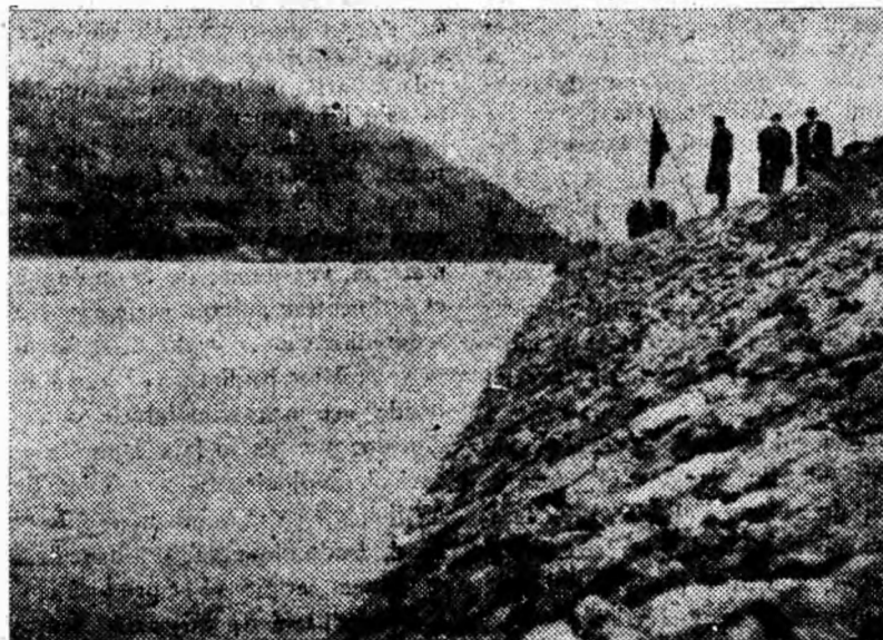
IN CLIȘEU: Apele vijelioase ale Jiului au pornit pe noua albie.
