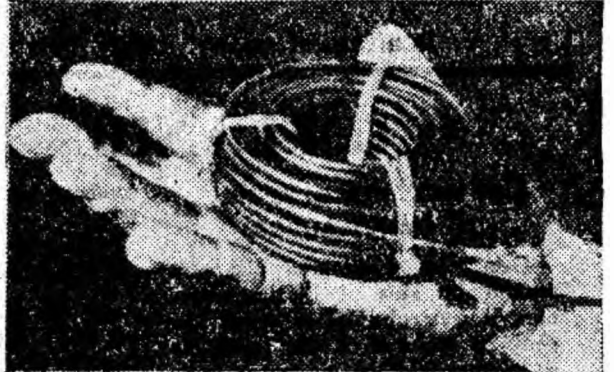
Diametrul noului cablu care se vede în fotografie este de 4,5 milimetri. Acest cablu este destinat cercetării geofizice a puțurilor de foraj. Blindajul cablului rezistă la o greutate de 600 de kilograme, iar stratul izolator suportă o tensiune de 1.650 de volți la o temperatură de 200°C.
