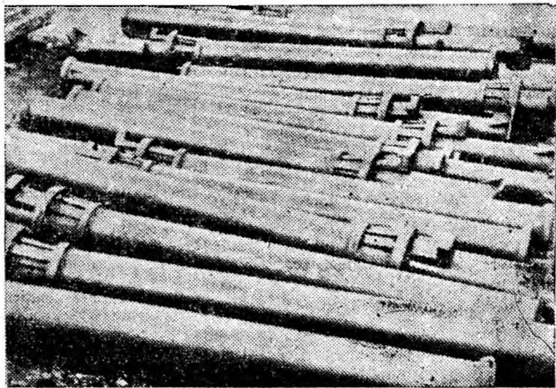
In prima jumătate a acestui an, un colectiv de ingineri și tehnicieni de la mina Petrila a realizat un sistem de susținere care folosește stâlpi cilindrici confecționați din tuburile degradate de la rambleu. Reluându-se și completându-se de către specialiștii de la C.C.V.J. inovația a fost îmbunătățită. La U.R.U.M.P. s-a confecționat de curând un lot experimental de stâlpi cilindrici pentru extinderea folosirii lor. IN CLIȘEU: Lotul experimental de stâlpi cilindrici gata pentru exploatarea la exploatare.
