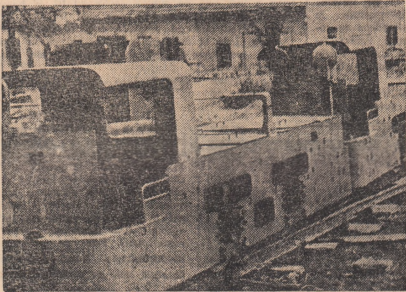
La mina Dilja sînt în curs de execuție lucrările pentru electrificarea transportului. Se instalează linia aeriană de curent continuu pe traseele principale de transport de la suprafață, au sosit locomotive electrice cu care se va efectua un transport mai rapid și mai economic. În fotografiile cele două locomotive electrice cu trolley sosite de curînd la mina Dilja.
