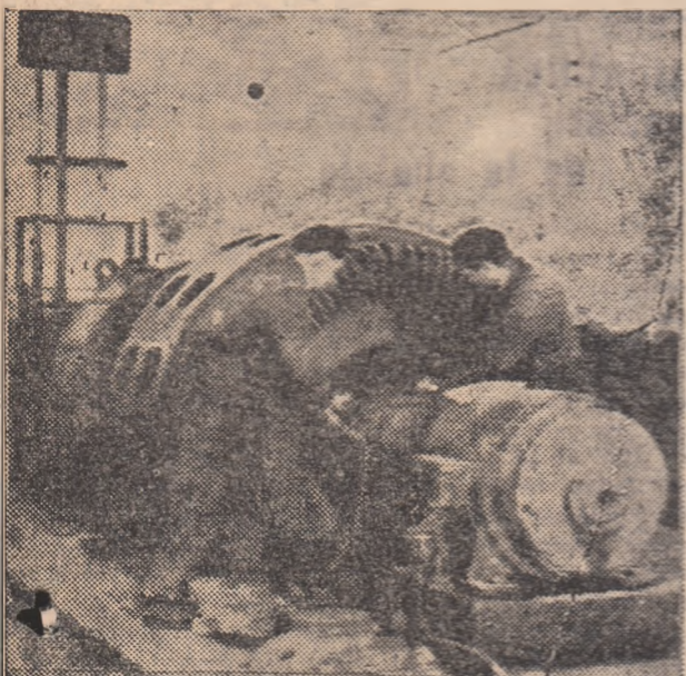
Una din lucrările importante executate în acest an de I.C.M.M. a fost construcția puțului 12 Lupeni. IN CLIȘEU: Electricienii Szabo Ștefan și Szilagy Iosif lucrînd la convertizorul noului puț al minei Lupeni.
