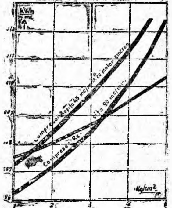
Variația consumului specific de energie electrică la compresare.
