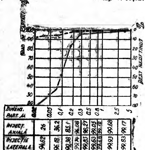
Fig. 2. Gradul de captare a perforajului umed de diverse fracțiuni de dimensiuni ale prafului.
