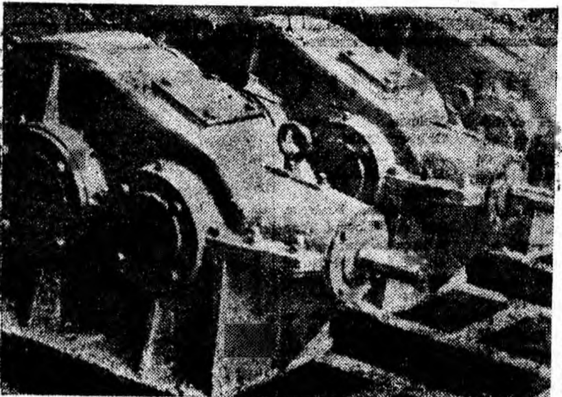
Lista utilajelor și pieselor de mașini produse în ultimul timp la U.R.U.M.P. cuprinde și un lot numeros de cutii de acționare pentru instalațiile de transport cu lanț elevator de la exploatarea miniere. IN CLISEU: Cîteva din aceste utilaje.
