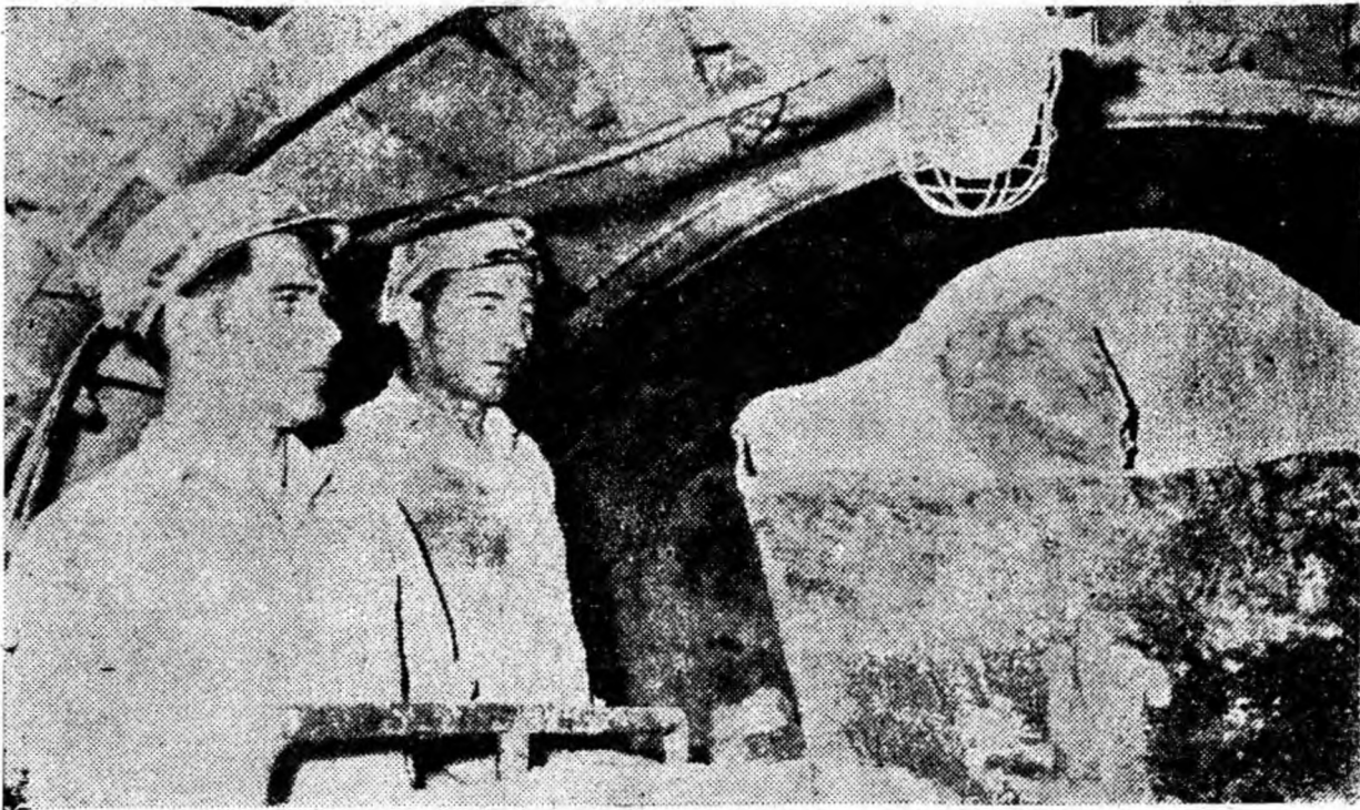
Minerul șef de schimb Ionașcu Ioan lucrând cu un ortac la încărcarea sterilului cu mașina electrică de încărcat E.P.M.-1.
