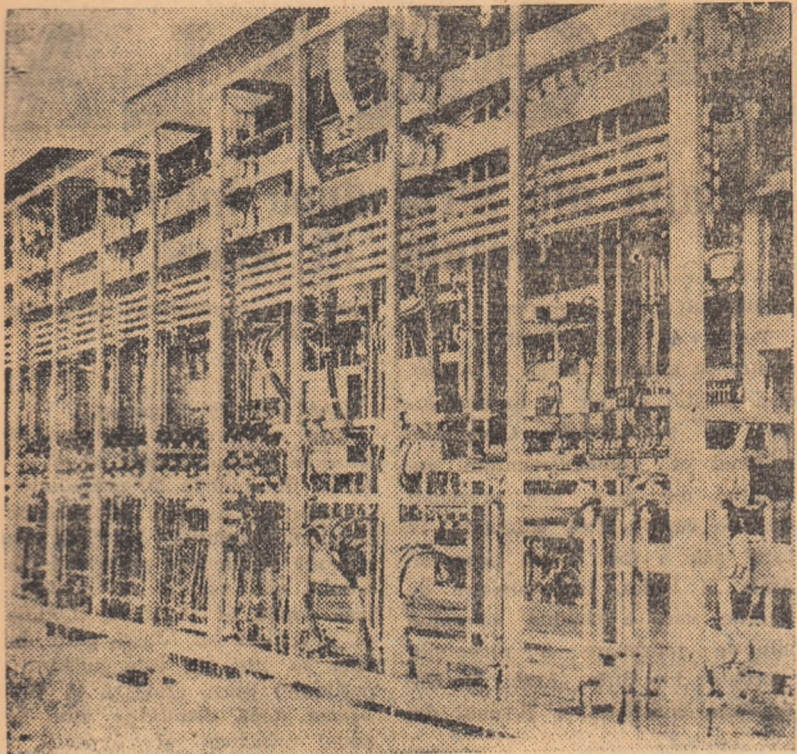
Mare și impunătoare, noua preparație de cărbune din Coroiști e înzestrată cu utilaje moderne de înaltă productivitate. O bună parte din comenzi sînt automatizate. În clișeu se pot vedea o parte din circuitele de la distribuitorii RM-5.
