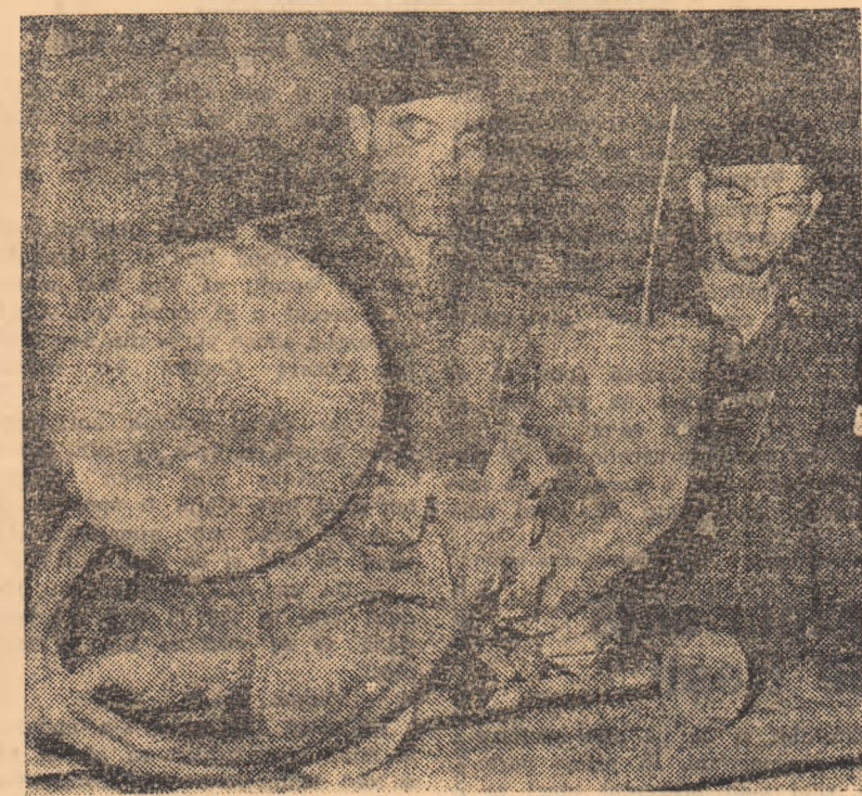
La U.R.U.M.P. se extinde continuu mecanizarea procesului tehnologic. Rezultate bune se obțin la sudarea automată a stîlpilor metalici de abataj. Prin utilizarea mașinii automate de sudat s-a scurtat la 46 de minute timpul de lucru pentru sudarea unui stîlp metalic G.H.H. față de 80 de minute cît ar fi necesar dacă sudarea s-ar face manual. ÎN CLIȘEU: Sudorii Pădureanu Constantin și Rotaru Antonie din secția construcțiilor metalice lucrînd cu mașina automată de sudat.
