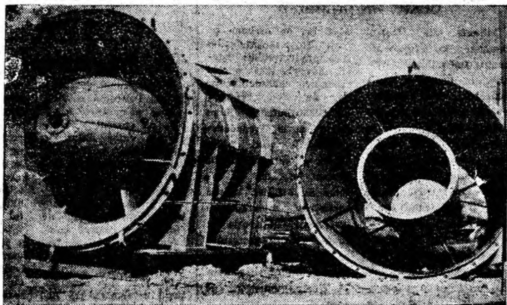
La mina Petrila se află în construcție noua stație de ventilatoare de la puțul est nr. 1. Stația va servi pentru intensificarea aerajului în partea estică a minei, respectiv blocul zero. În clișeu poate fi văzut unul din cele două ventilatoare axiale tip V.O.K.D.1,8 de fabricație sovietică, cu care va fi echipată noua stație de ventilatoare.
