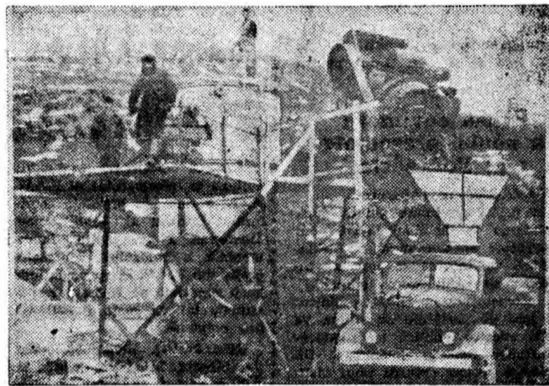
3) Stația de preparare a betonului.
