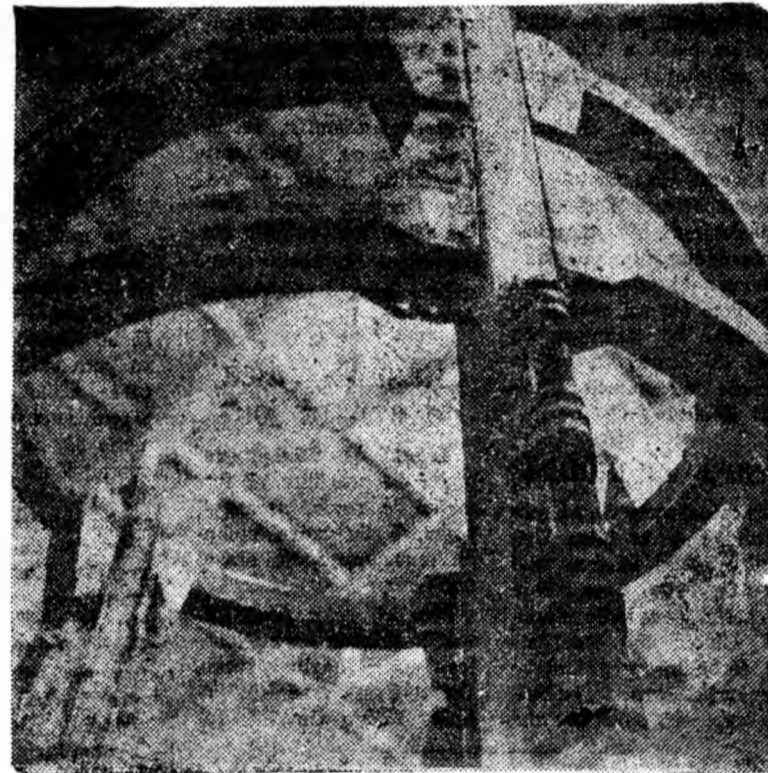
La secția construcții metalice de la U.R.U.M.P. se confecționează un nou cofraj mobil de 4 m pentru săparea puțurilor de mină.
