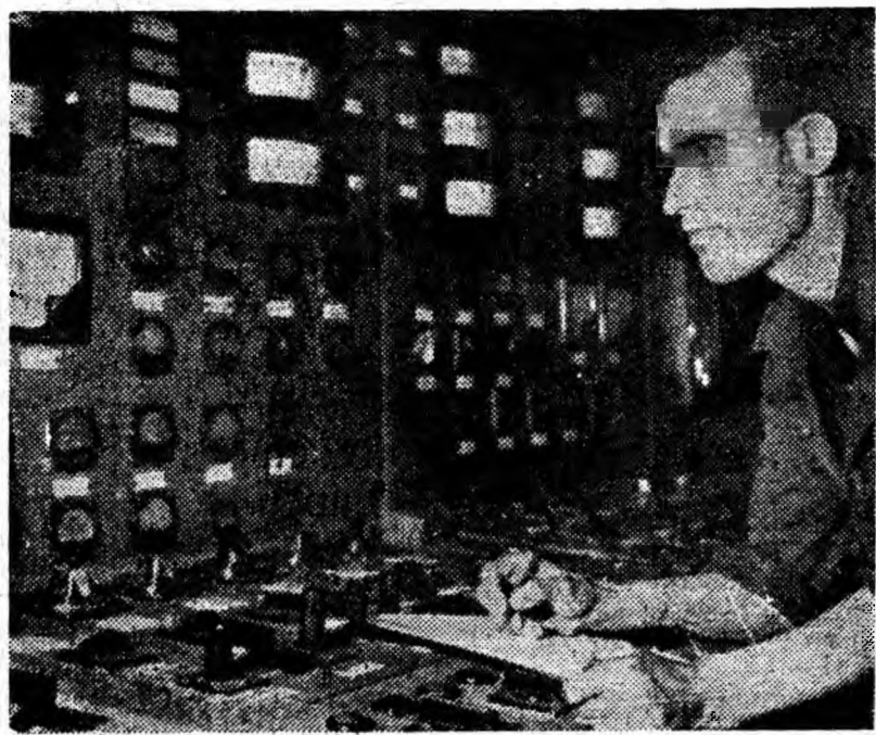
Mechanicul principal Munteanu Ilie, din secția cazane, este unul dintre cei mai buni muncitori de la termocentrala Paroșeni. Clișeul îl înfățișează în timp ce urmărește parametrii cu care funcționează cazanul, care sînt indicați de aparatele de pe tablou.
