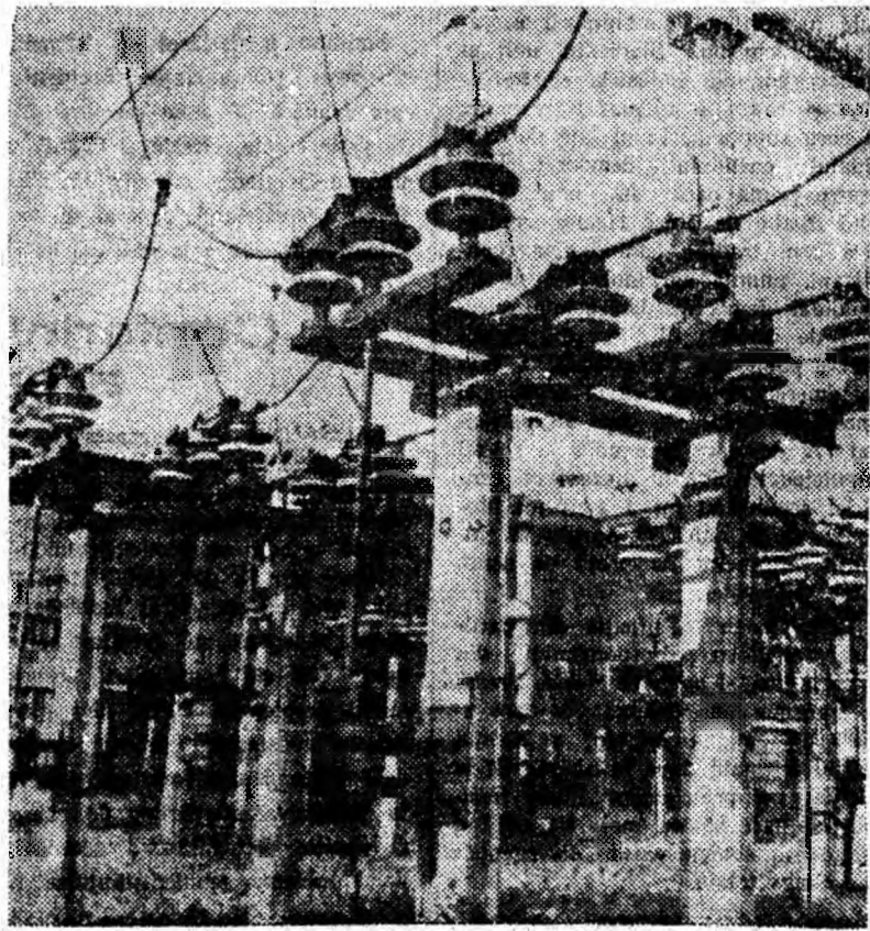
În clișeu de față vă prezentăm o parte din instalațiile stației de transformare de la Fero. De aici, prin firele de înaltă tensiune, curentul electric își ia drumul spre adîncurile minel Petrița și spre preparate
