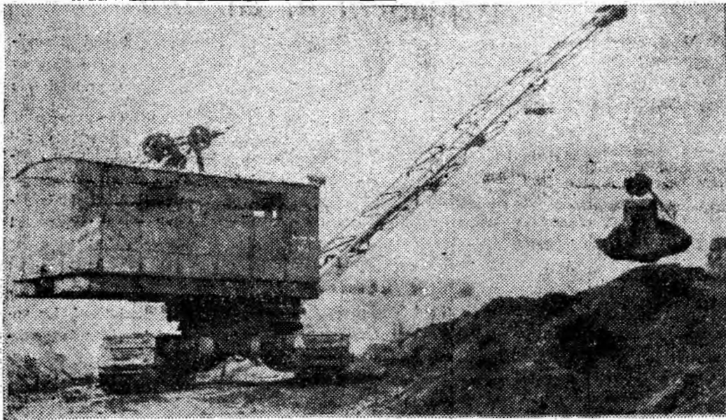
PAROȘENI. Zilnic, pe rampa termocentralei sosesc cantități însemnate de cărbune. Iată macaraua greifer lucrînd la stocarea lui.
