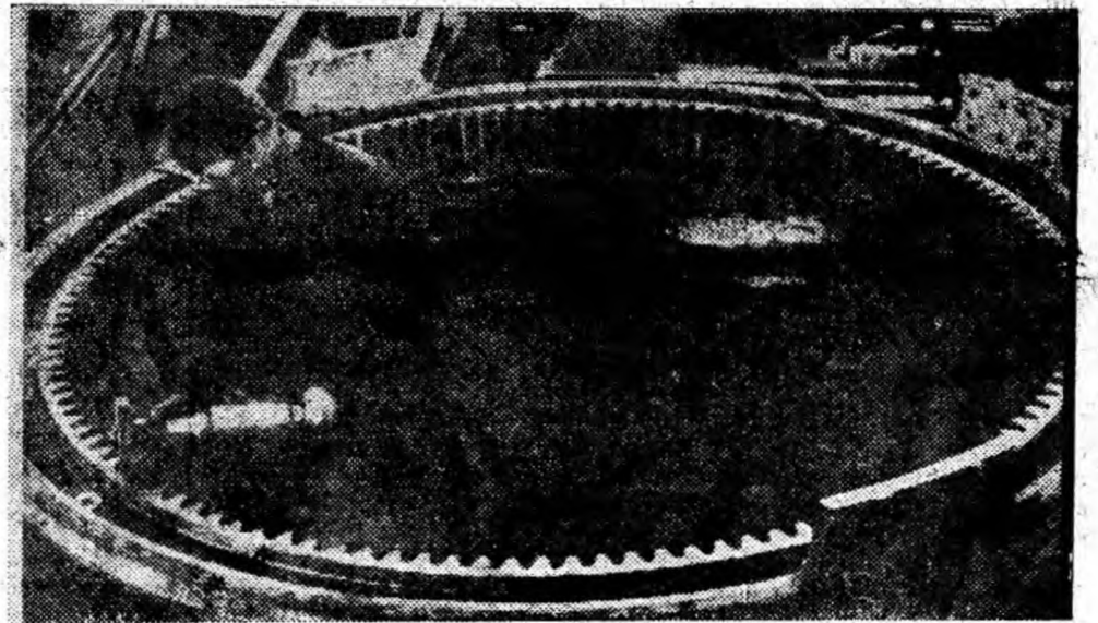
Secția mecanică, U.R.U.M.P. Aici, piesele — roți, axe, pinioane, bușe, lagăre — sînt prelucrate, primindu-și forma definitivă, înainte de a lua drumul către exploatare și parașii. ÎN CLISEU: Polizarea unei coroane dințate.
