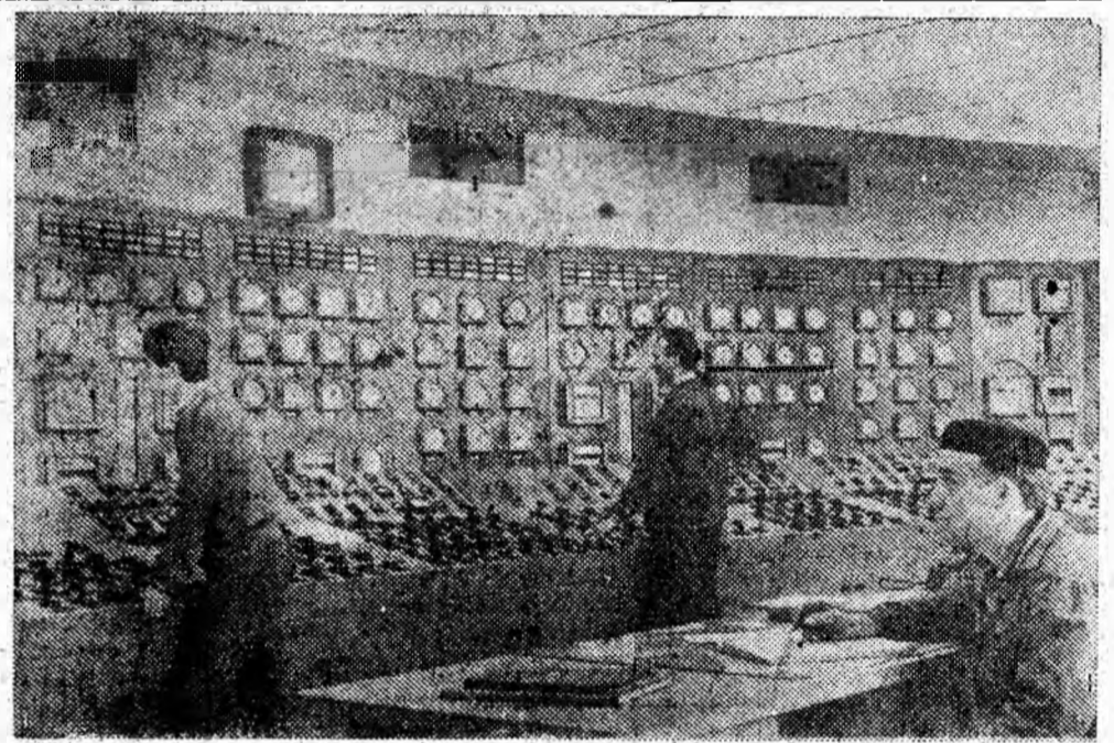
Sala de comandă termică a noului grup electrogen de 150 MW de la T. C. Petroșani.
