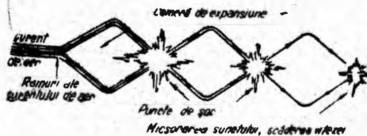
Fig. 2. Schema funcționării amortizorului de zgomote.
