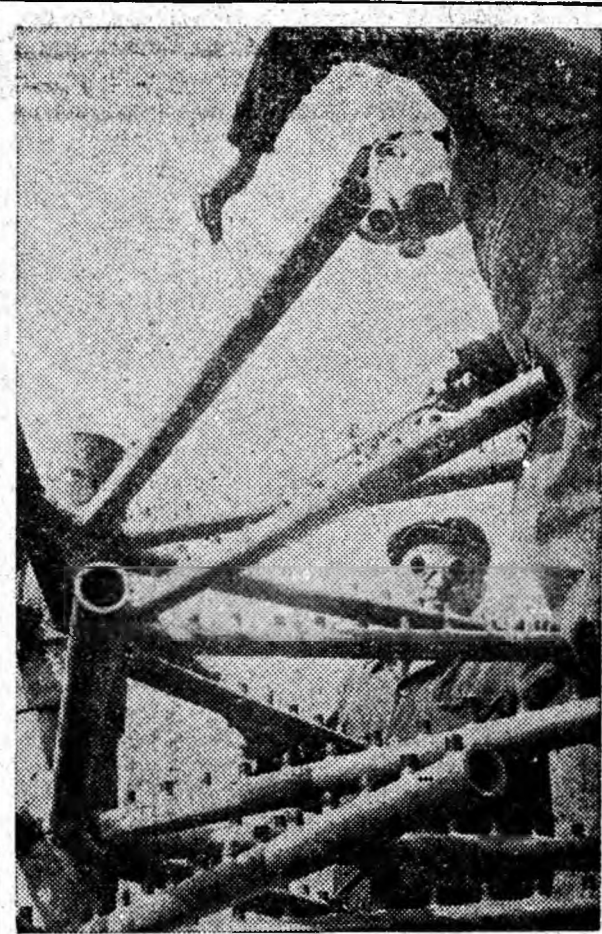
Sudorul Capriș Vasile și lăcătușul Szasz Alexandru de la Viscoza-Lupeni execută un dispozitiv pentru filtrarea apei sub presiune. Cu ajutorul acestei instalații se îmbunătățește calitatea firelor produse.
