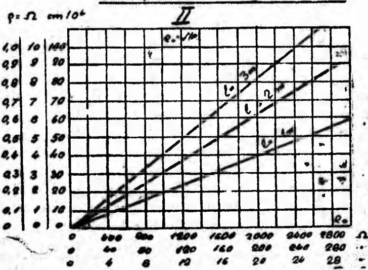
Pentru prize definitive îngropate la 1 m sub nivelul solului țevi \phi 2'' l = lungimea țevii.
