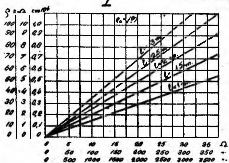
Pentru prize definitive îngropate la 1 m sub nivelul solului țevi \phi 2'' l = lungimea țevii.
