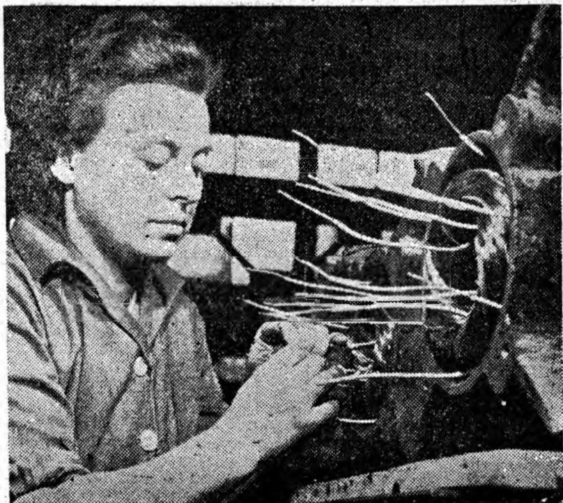
Bobinatoarea Iler Maria, evidențiată în întrecere, de la S.R.E. Vulcan, executînd legăturile unui motor de 1,1 kW.
