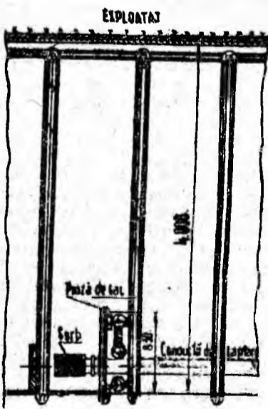
Rambleerea și exploatarea supra-puse în abatajele cameră din stratul 3.
