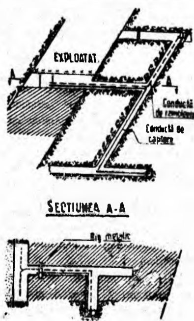
Montarea digului metalic.
