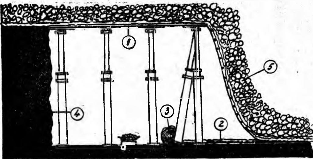
1. Tavanul artificial din rețea de cabluri și plasă metalică. 2. Noua poditură care se așterne pe vatră. 3. Sul de plasă metalică care urmează să fie desfășurat pe direcția frontului. 4. Frontul de lucru. 5. Spațiul exploatat înspre surpare.
