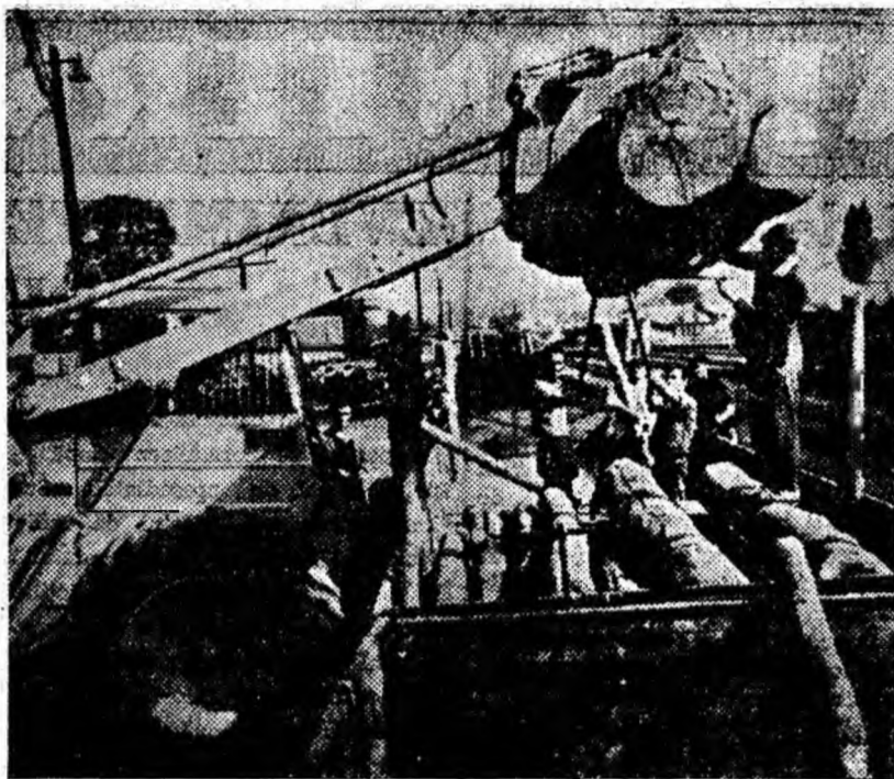
Pe rampa de la Lupeni, încărcarea buștenilor în vagoane se face cu mijloace mecanizate.
