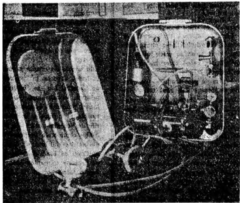
Aparat de salvare tip Medl, folosit la exploatarea miniere din Valea Jiului.
