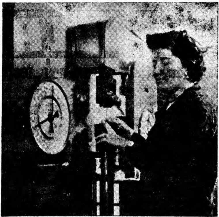
Laboratorul mecanic de la U.R.U.M.P. Se încearcă rezistența la rupere a firelor de la cablurile de extracție.
