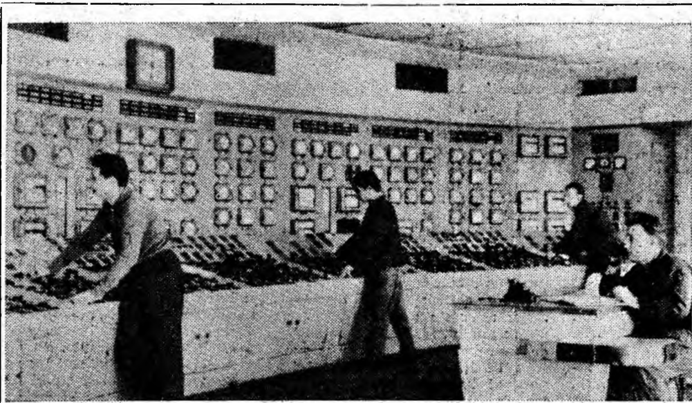
Aspect din camera de comandă a grupului electrogen de 150MW/h de la I.E.C. Petroșani
