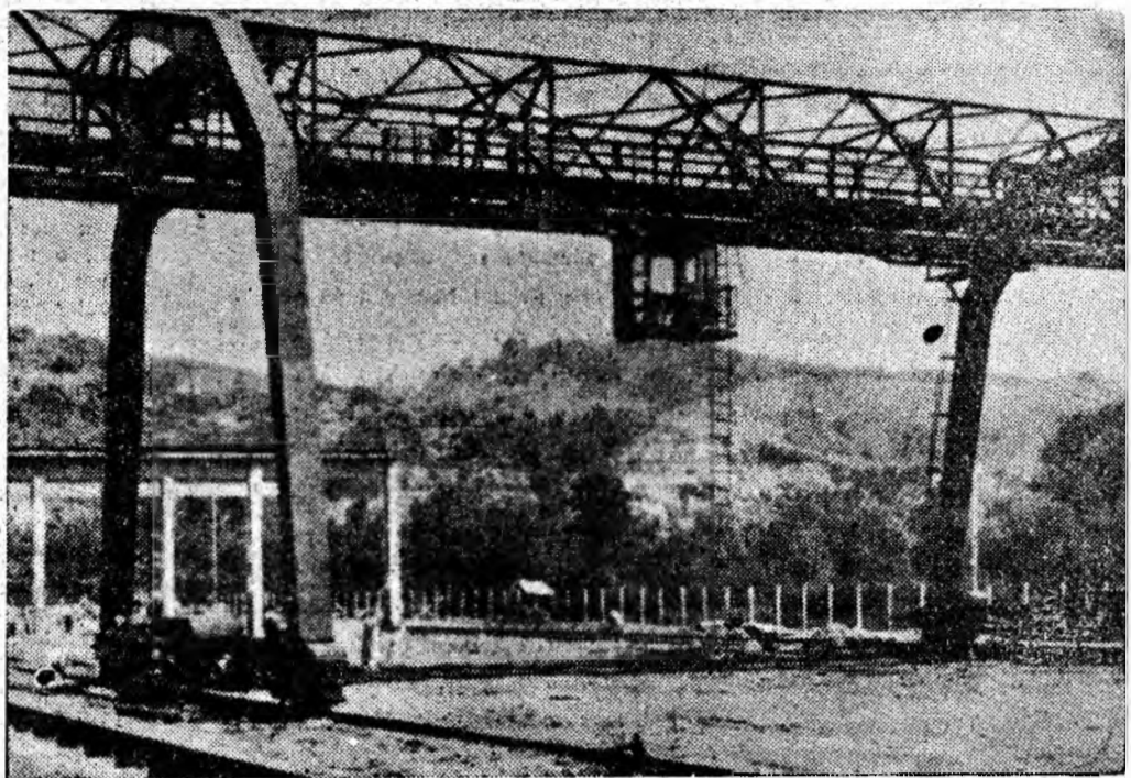
La Aninoasa sud, sînt pe terminate lucrările la noul depozit de materiale. Operațiile de încărcare-descărcare a materialelor din vagoane vor fi mecanizate cu ajutorul podului rulant montat în incinta depozitului (în fotografie).
