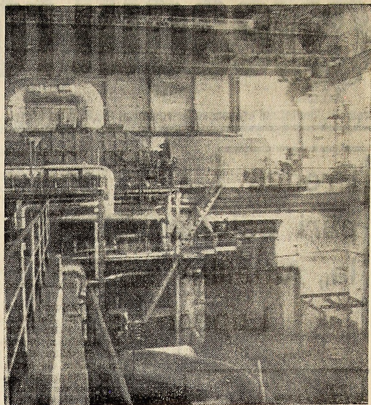
Aspect din sala de turbine a grupului nr. 4 de la Termocentrala Paroșeni.
