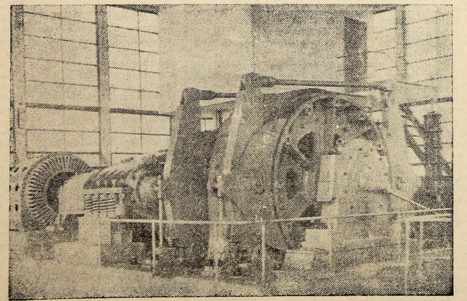
Puternicele motoare care acționează la pușul cu schip de la muna Lonea.
