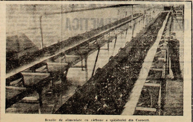
Benziile de alimentare cu cărbune a spălătoriei din Coroesti.
