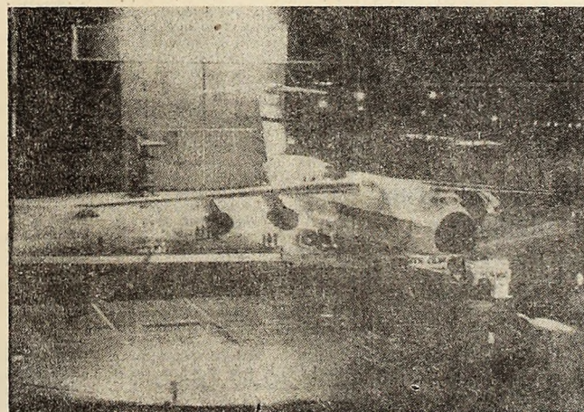
S.U.A. Cel mai mare avion din lume, construit de societatea Lockheed-Georgia U.S.A., va fi supus ultimelor probe la baza aeriană din Dobbins. ÎN CLISEU: Ieșirea din hangare a avionului „C-5 Galaxy” care are o anvergură de 67 m și o lungime de 74 m.
