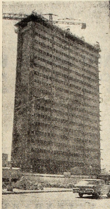
REPUBLICA CUBA: Această impunătoare construcție, amplasată pe una din străzile Havanei, a fost înălțată într-un timp, socotit record de construcții cubaneze, datorită folosirii panourilor prefabricate. Construcția are 17 etaje și o înălțime de 55 m.
