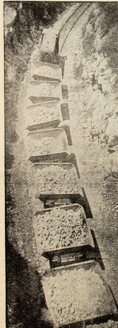
BĂNIȚA. „Cupele” cu calcar în drum de la carieră spre rampa de descărcare.
