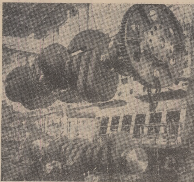
R.P. POLONA: Hala de montaj a motoarelor la fabrica „Gegielski” producătoare de locomotive și vapoare.
