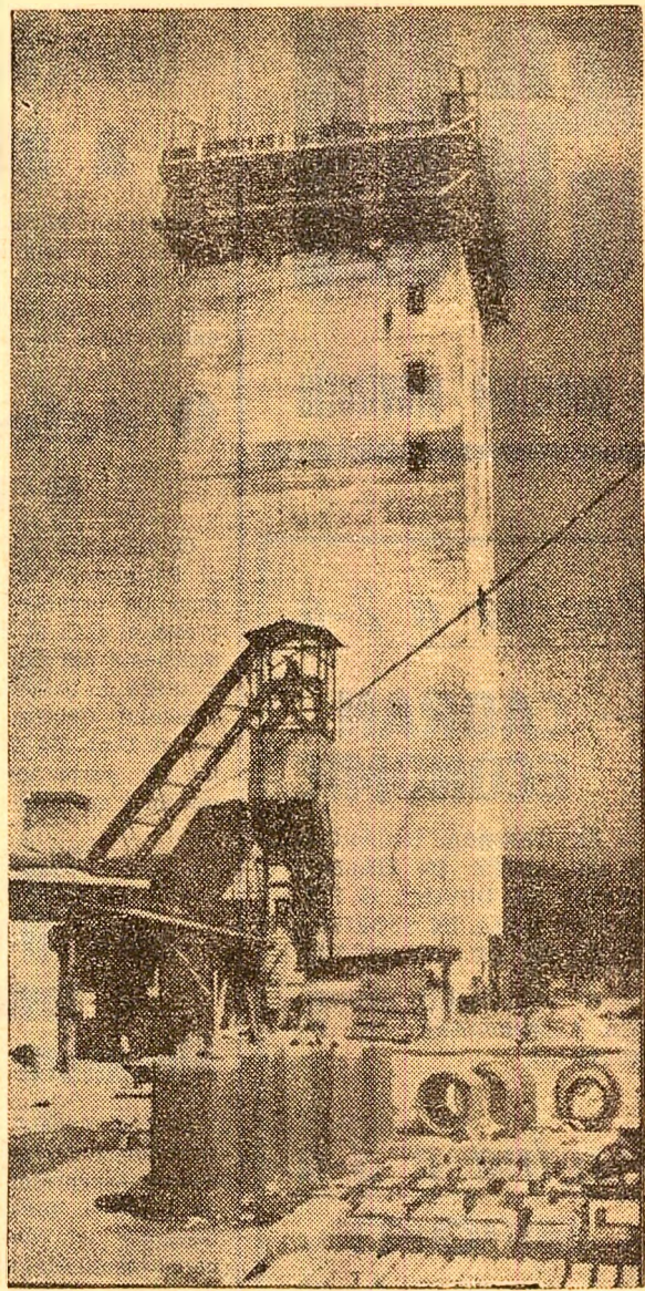
O nouă siluetă arhitectonică în peisajul Petroșaniului: turnul puțului minei Livezeni — lucrare aflată în plină glisare.
