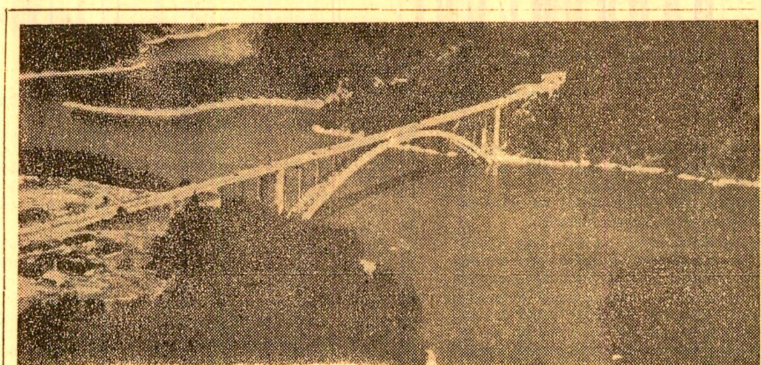
R. S. Cehoslovaca. — Podul din satul Zdanov, Boemia, construcție de oțel de 570 m lungime cu un arc de deschidere de 330 m.
