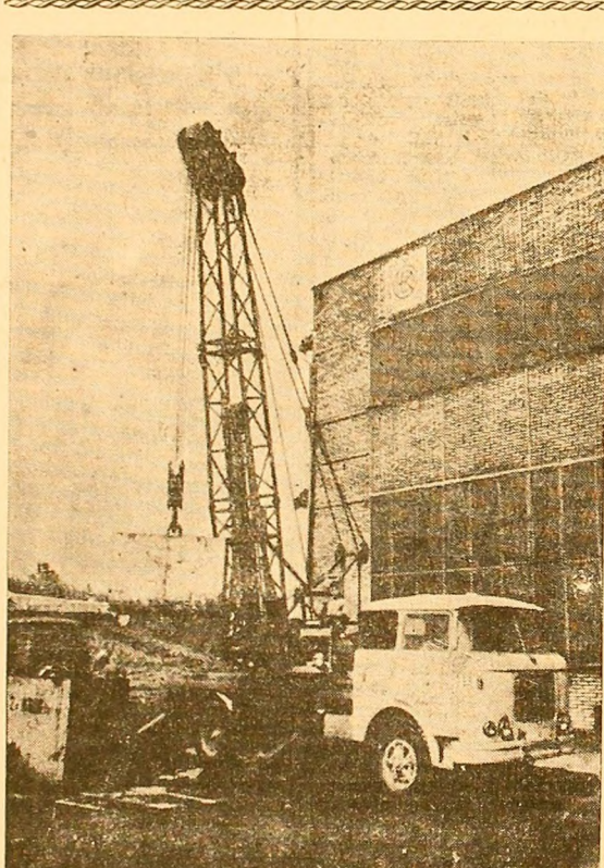
R. S. CEHOSLOVACA: Macara mobilă AD-100 cu o capacitate de ridicare de 10 tone greutate, construită recent în Cehoslovacia.
