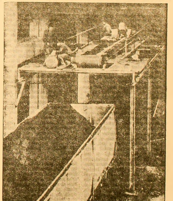
Preparația Coroșei: Se efectuează ultimele lucrări de montare la benzile de planșare a cărbunelui în vagoanele de pe linia a-3a.
