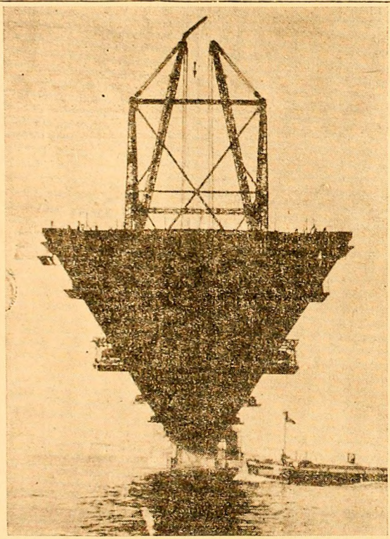
R. F. a GERMANIEI: Un nou pod peste Rin, la Düsseldorf, este în construcție. Podul va fi terminal la sfârșitul anului 1969 și va uni cartierul Oberkassel cu centrul orașului.
