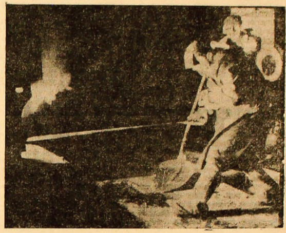
U.R.U.M. Petrosani. La secția turnătorie a uzinei se elaborează o nouă șarjă de oțel necesar turnării pieselor folosite pentru reparatiile efectuate la uzilele miniere.
