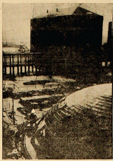
R. P. UNGARĂ: Secțiune a clădirii reactorului atomic de pe lângă Universitatea Tehnică din Budapesta. Clădirea se află în faza finală de construcție.
