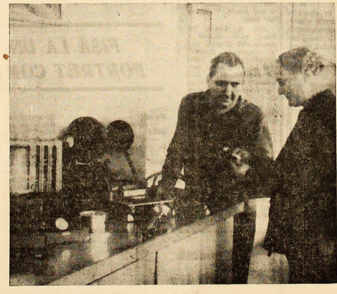
Aspect din laboratorul de aeraj al S.C.S.M. Petroșani. Inginerul Alexandru Dicu și tehnicianul Iosif Budau verifică aparatul pentru determinarea condițiilor climatice din subteran.
