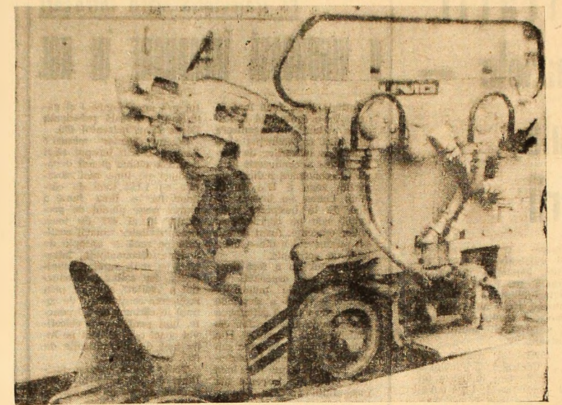
Prezență devinită obișnuită în viața cotidiană a minierilor din bazin: mașinile de încărcare steril pentru lucrările de înaintare. Fabricate la Uzinele UNIO din Satu Mare, aceste mașini acționate cu aer comprimat sînt de un real sprijin pentru minierii de la înaintări înlocuindu-le muncă fizică grea la încărcarea sterilității.
