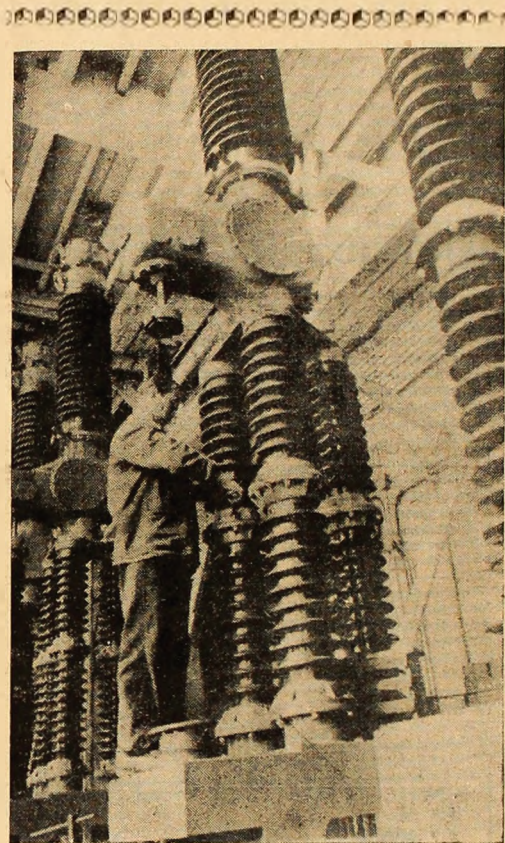
Asamblarea unei unități de circuit de mare capacitate la întreprinderea de aparate electrice de la Budapesta.
