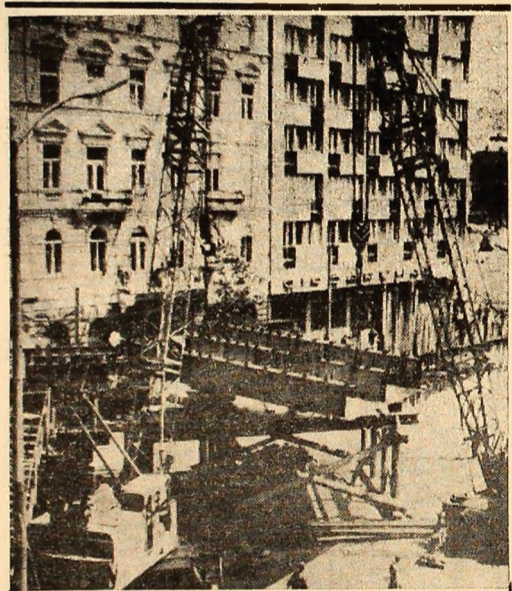
R. P. UNGARĂ. În cadrul lucrărilor de modernizare pe principalele artere din Budapesta se construiește o șosea suspendată în piața Boreas.
