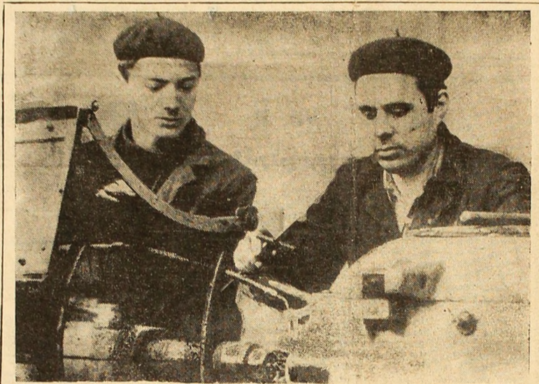
Strungarul Gal Ion, secondat de ucenicul Dragoș Vasile, strunjește „corpul ventilului” pentru stâlpii hidraulici — tip Sah. Foto: I. LICU
