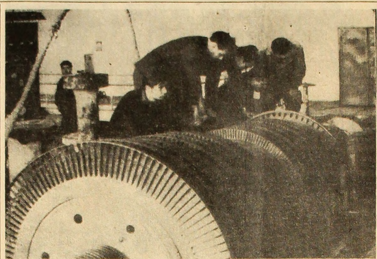
Termocentrala Paroșeni: Se lucrează la reparația planificată a corpului de înaltă presiune de la turbina de 150 megawați. Foto: I. LICIU
