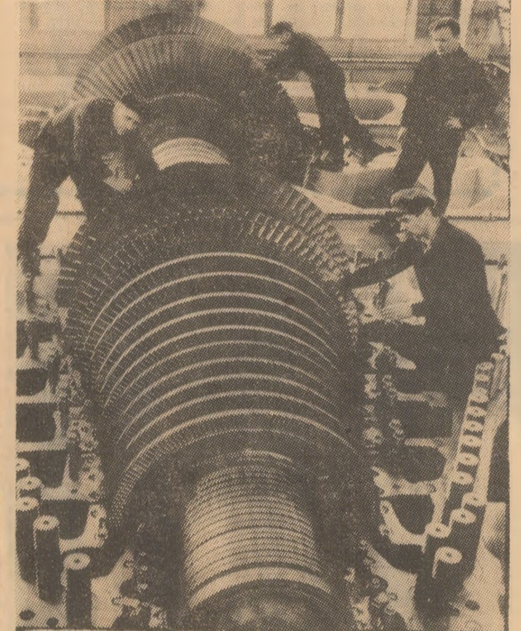
U.R.S.S.: Turbina VT 100 pregătită pentru livrare către beneficiar la Uzina de turbomotoare „Urali” din Sverdlovsk.
