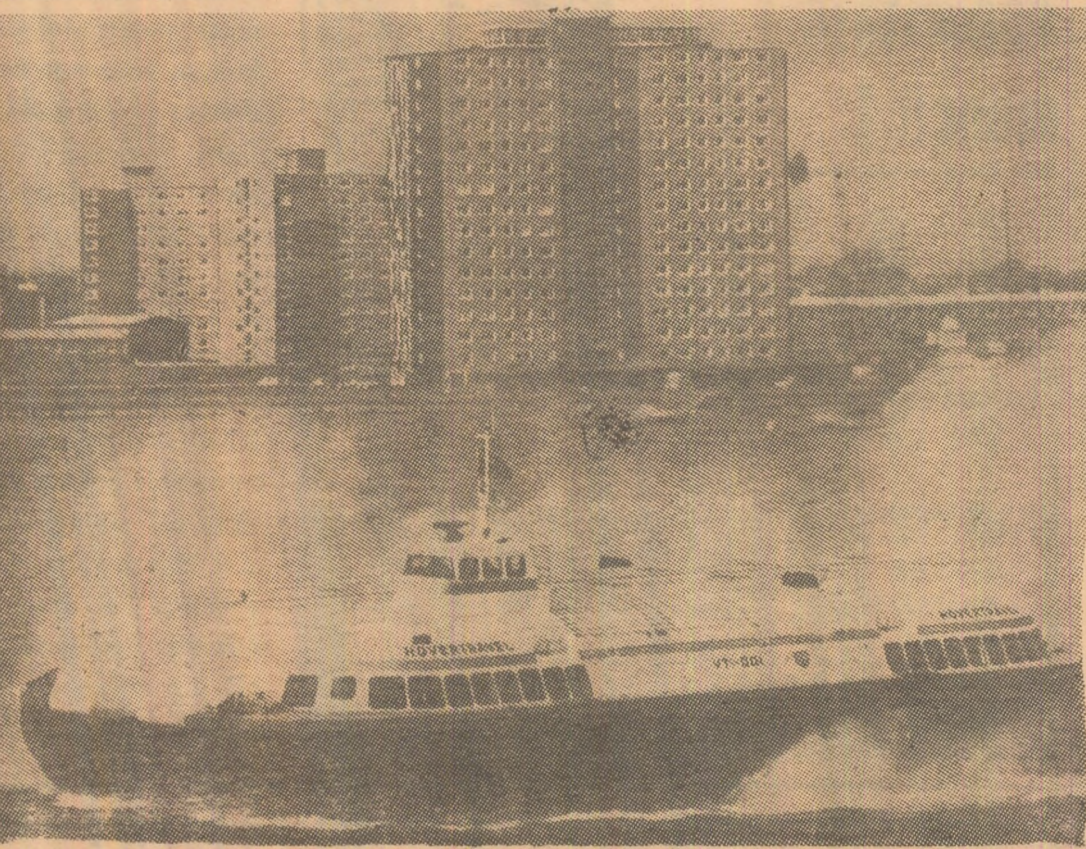
ANGLIA: Ambarcațiunea pe pernă de aer VTI-001, creată la Vesper Thornycroft, este primul vas din lume semi-amfibie. Seria standard cea din foto, poate transporta 146 de pasageri și 10 automobile. Pasagerii stau în patru saloane largi iar au o cabină într-un garaj central. Ambarcațiunea are o lungime de aproximativ 30 de m și o lățime de aproximativ 15 m și o viteză de croazieră de 40 de noduri.
